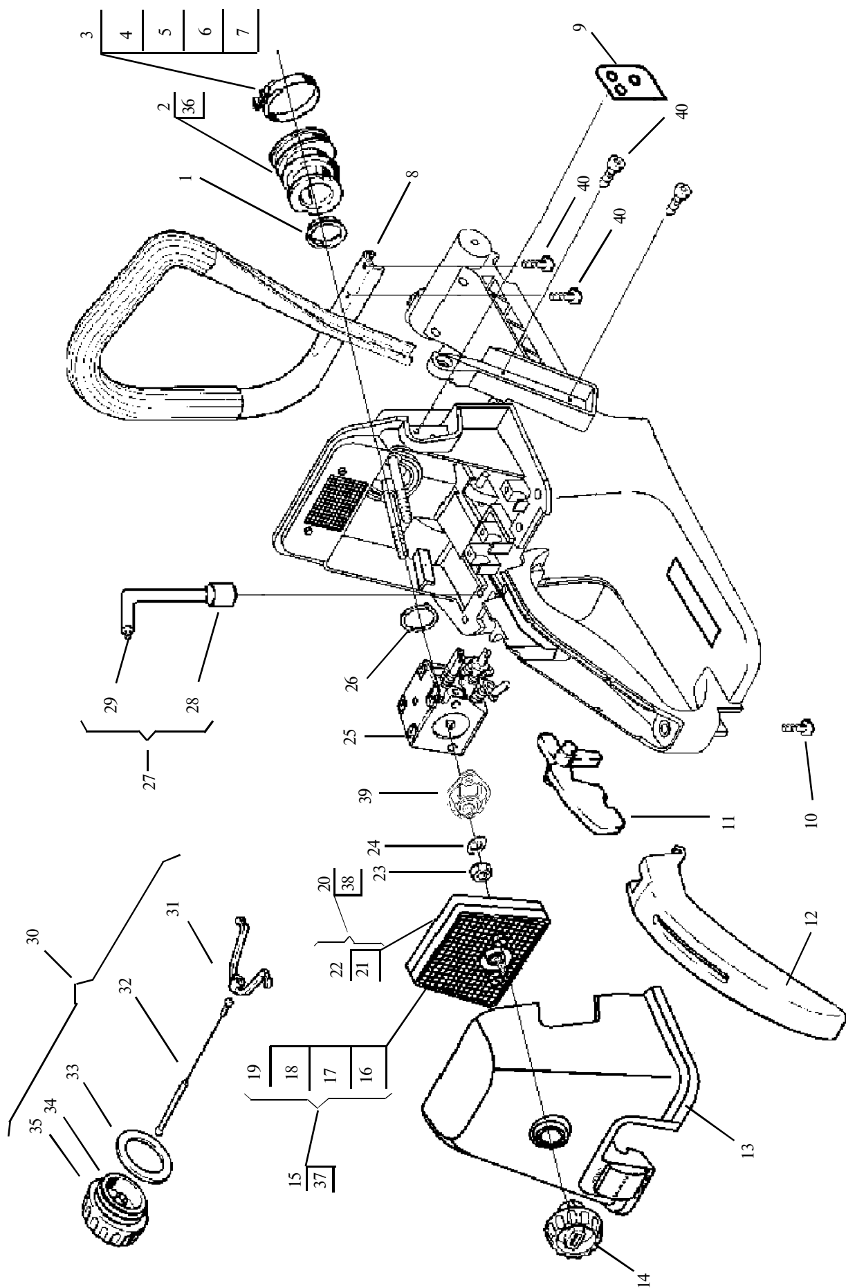
Рисунок 1.6 - Корпус-бак, карбюратор, воздушный фильтр
