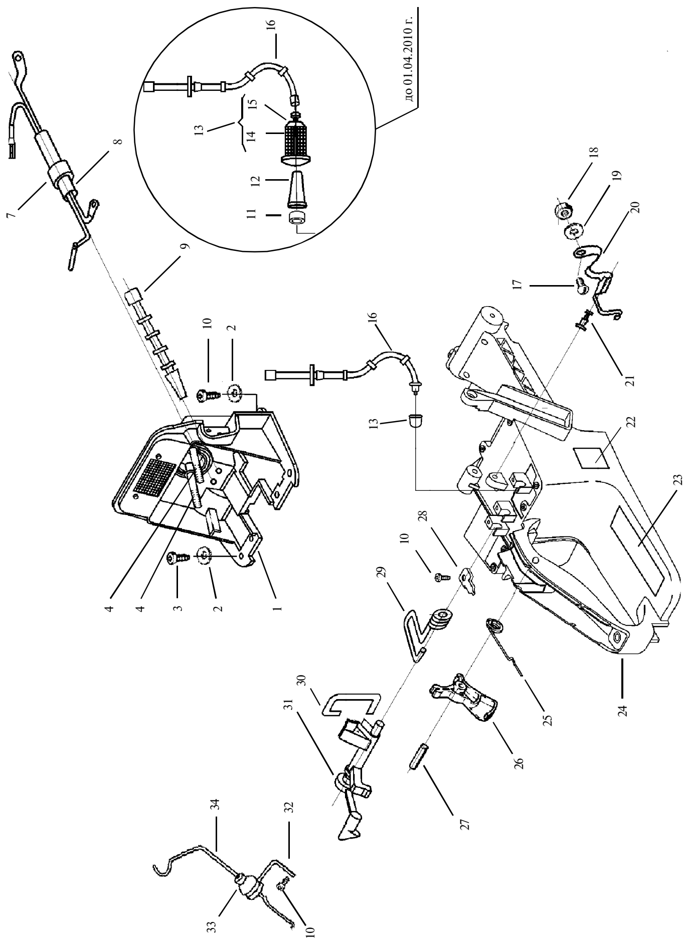
Рисунок 1.5 - Корпус-бак бензопилы
